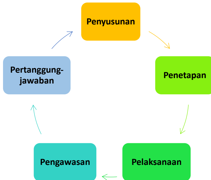
Gambar 1 Siklus APBN
